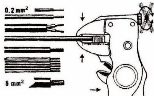
Art. Nr.: 9110 ABISOLIERZANGE
